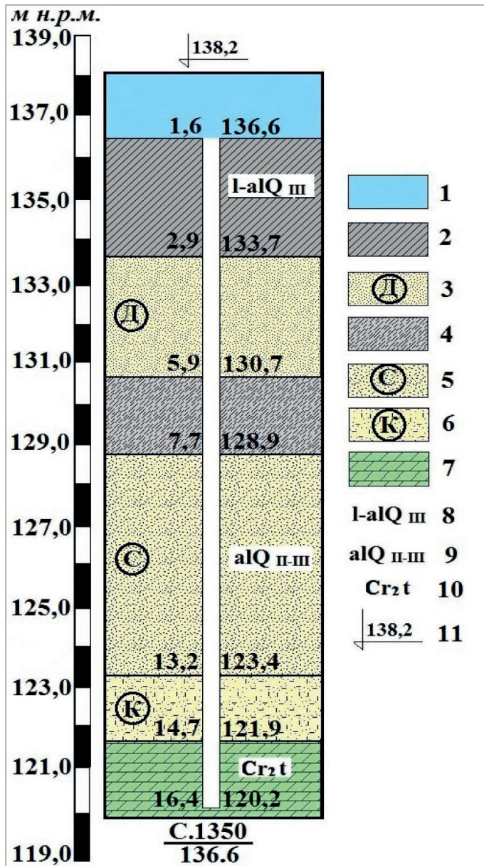
Рис. 4. Геологічна свердловина у центральній частині акваторії оз. Липенське (побудована за фондowymi матеріалами НДІ «Рівнедніпроводгосп»)
